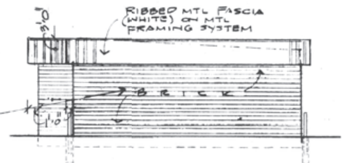
RIGHT SIDE ELEV.
