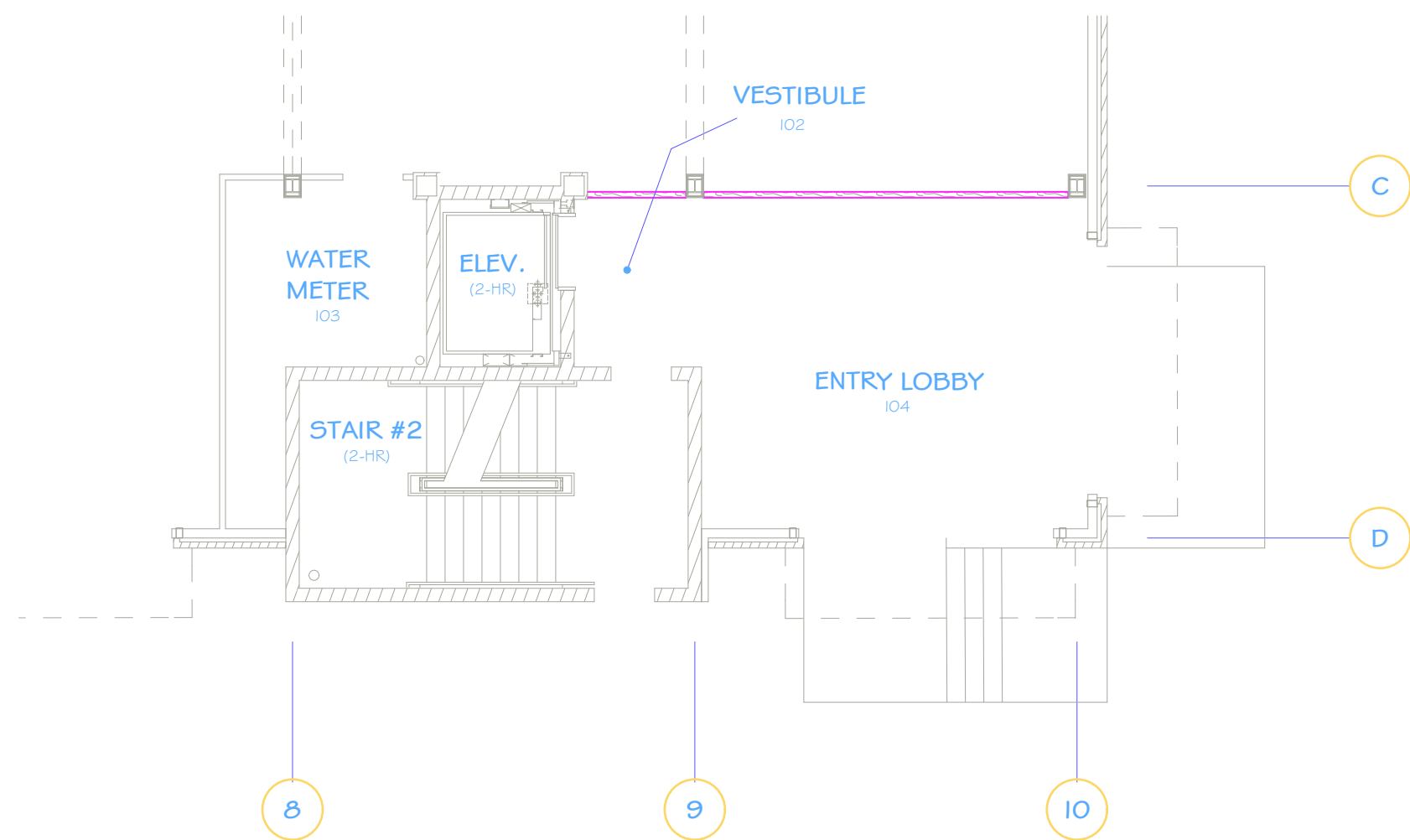
SCALE: 1/8" = 1'-0"
